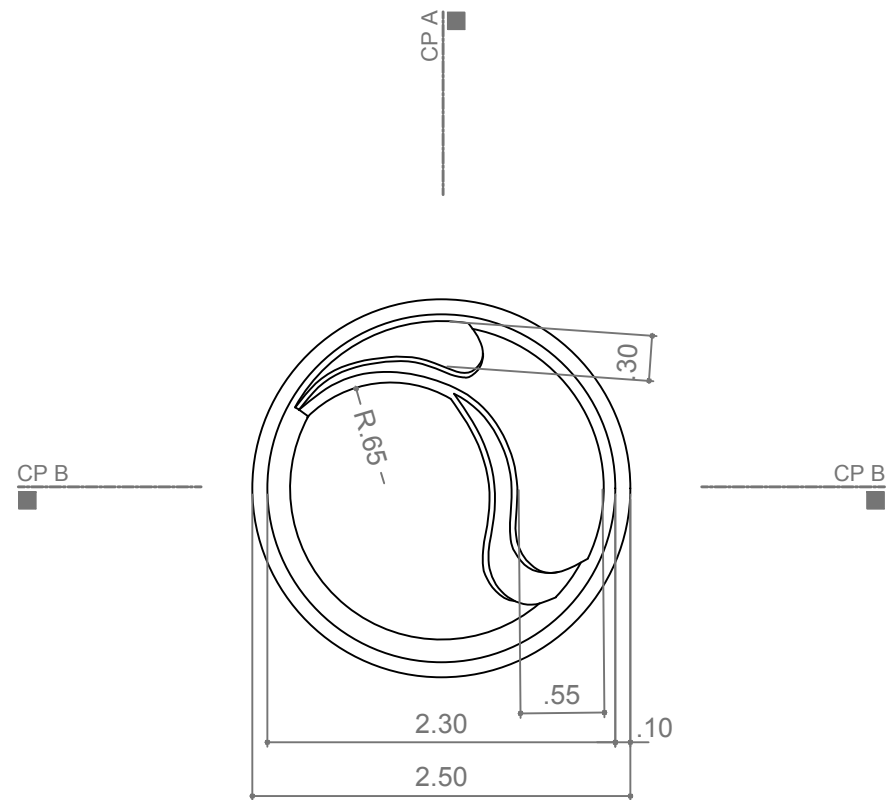
PLANTA BAIXA
