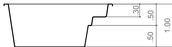
CORTE B
