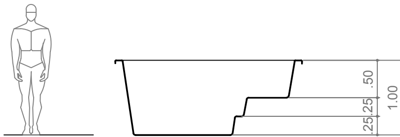
CORTE A
